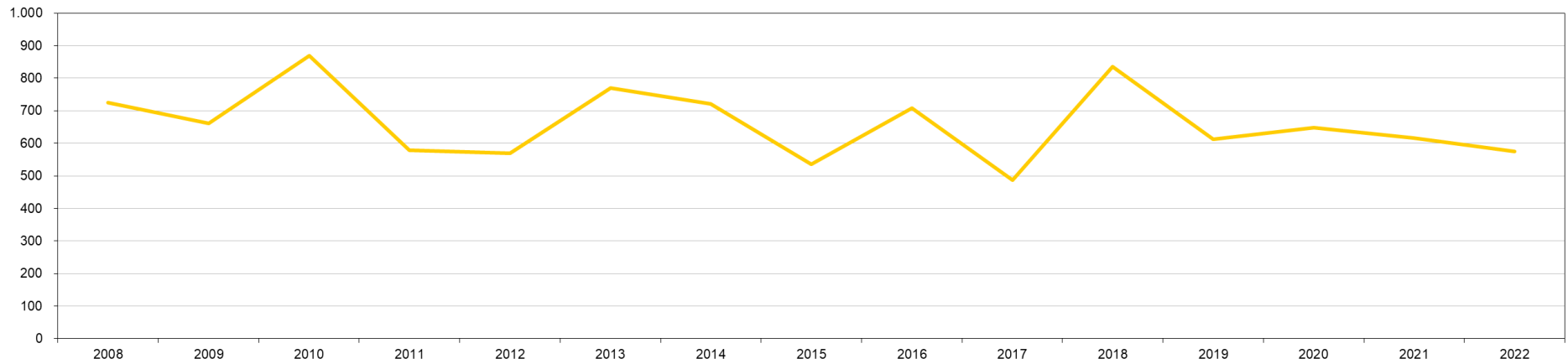
GRÁFICO 1: Evolución de la precipitación media (milímetros)
